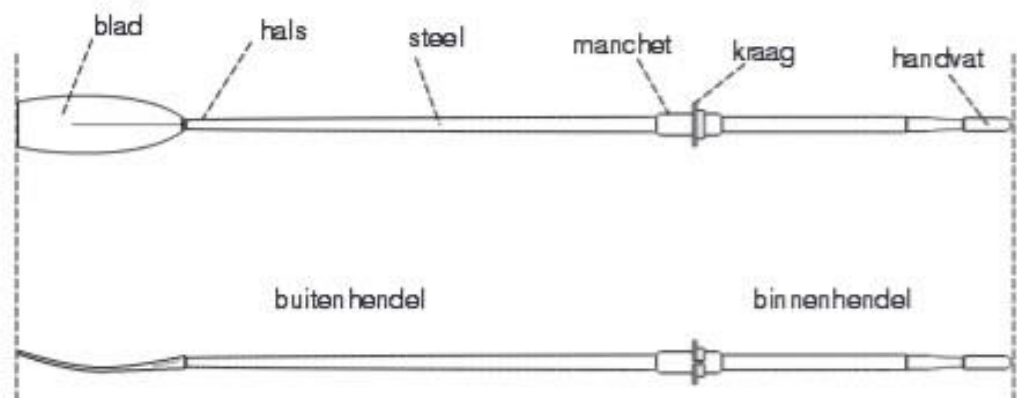
Afbeelding 5 Onderdelen van een riem
