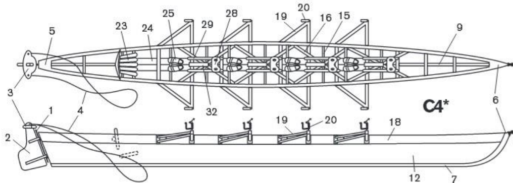
Afbeelding 1 Onderdelen van een boot, boven- en zijaanzicht
